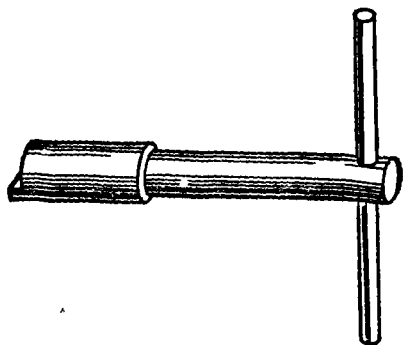
10. Оправка для снятия распределительного вала из картера двигателя
