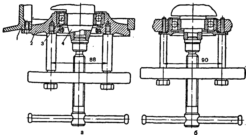
Р и с. 33. Выпрессовка кривошипного механизма или коленчатого вала универсальным съёмником:
