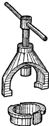
20. Съемник подшипника с задней цапфы коленчатого вала
