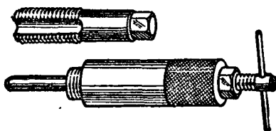
47. Съёмник с метчиком для демон- тажа седла клапана
