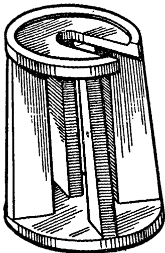
60. Приспособление для снятия ше- стерни четвертой передачи с веду- щего вала
