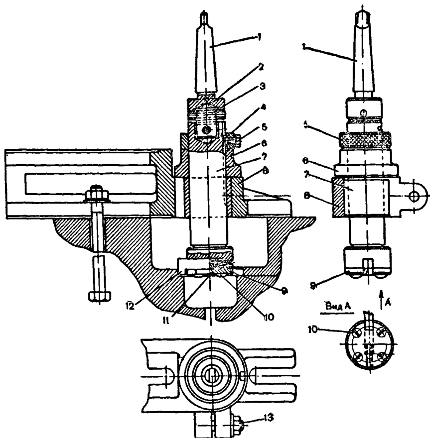
Рис. 44. Приспособление для расточки под седло клапана:
