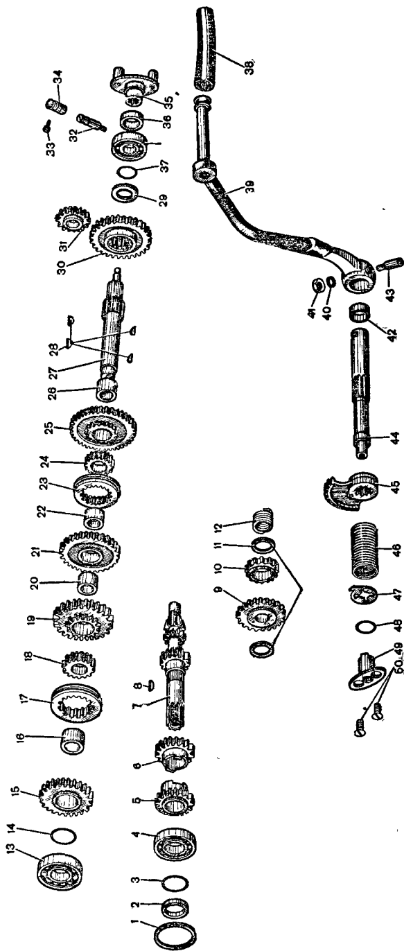
Рис. 53. Ведущий и ведомый валы и пусковой механизм коробки передач МТ-804 в разобранном виде: 1, 2, 3, 48 — кольца; 11, 14, 29, 37, 40 — шайбы; 4, 13, 30 — шарикоподшипники; 5, 6 — зубчатые колеса третьей и четвертой передач ведомого вала; 7 — ведущий вал; 8 — шпонка; 9, 10 — зубчатые колеса пускового механизма; 12, 46 — пружины; 15, 19, 21, 24 — зубчатые колеса четвертой, третьей, второй и первой передач ведомого вала; 16, 42, 49 — втулки; 17, 22 — муфты переключения; 18, 23 — муфты ведомого вала; 20, 28 — втулки; 26 — ведомый вал; 27 — шпонка; 28 — зубчатое колесо заднего хода ведомого вала; 31 — передаточное зубчатое колесо заднего хода; 32 — зубчатое колесо спидометра; 33 — болт; 34 — втулка зубчатого колеса спидометра; 35 — диск; 36 — ведущее зубчатое колесо спидометра; 38 — резиновая втулка; 39 — рычаг пускового механизма; 41 — гайка; 43 — клиновидный болт; 44 — вал пускового механизма; 45 — винты крепления втулки вала пускового механизма; 50 — упорная шайба; 47 — винт крепления сектора; 41 — винт крепления втулки вала пускового механизма
