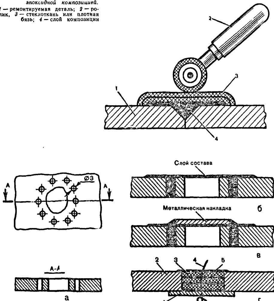
Рис. 2. Схема заделки эпоксидной композицией пробоин.
