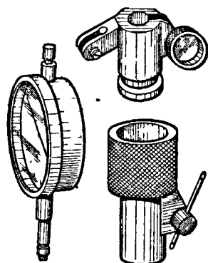
45. Приспособление для проверки концентричности фаски седла клапана
