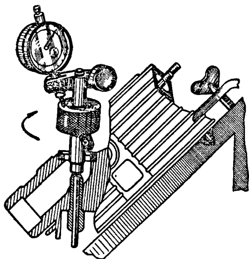
Рис. 29. Приспособление для проверки concentricности седла клапана с направляющей втулкой
