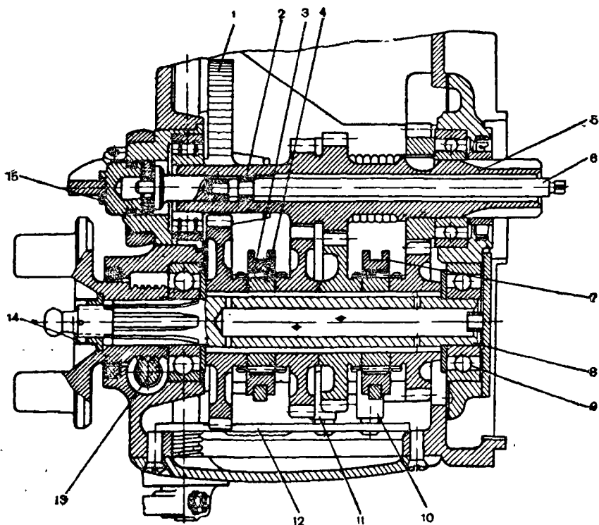
Р и с. 48. Коробка передач 6204 (разрез по валам);
