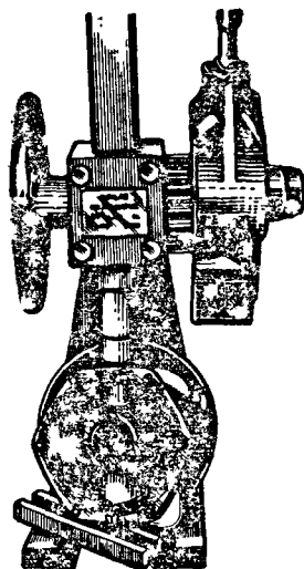
Р и с. 60. Запрессовка и выпрессовка деталей главной передачи
