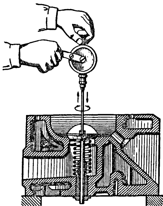
Рис. 30. Притирка клапанов с помощью дрели
