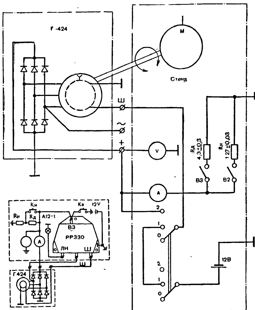
Рис. 68. Электрическая схема генератора Г-424 и реле-регулятора РР-330; Рд—5,73 Ом; Rн—1,27 Ом; А12-1—лампа; Кн—кнопка нагрузки; Кв—кнопка включения аккумуляторной батареи; справа представлена схема проверки генератора на стенде
