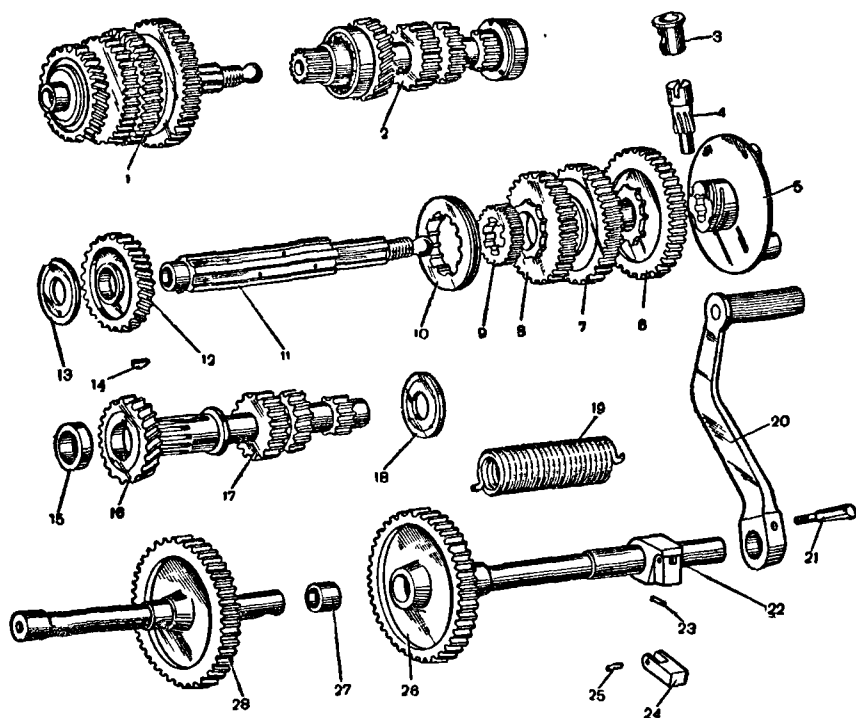
Рис. 50. Вали и зубчатые колеса коробки передач мотоциклов «Урал»:
