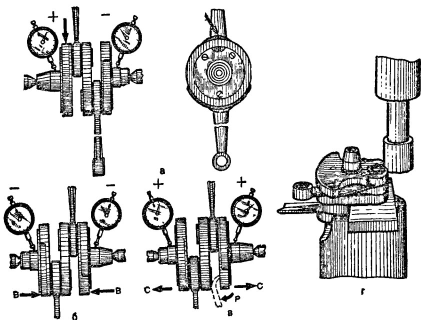
Рис. 37. Проверка и правка коренных шеек кривошипного механизма: а — с помощью оправки и индикатора; б — то же с разворотом на 180^\circ ; в — то же с разворотом на 180^\circ при плюсовых индикаторах; г — с помощью рычага или прессы
