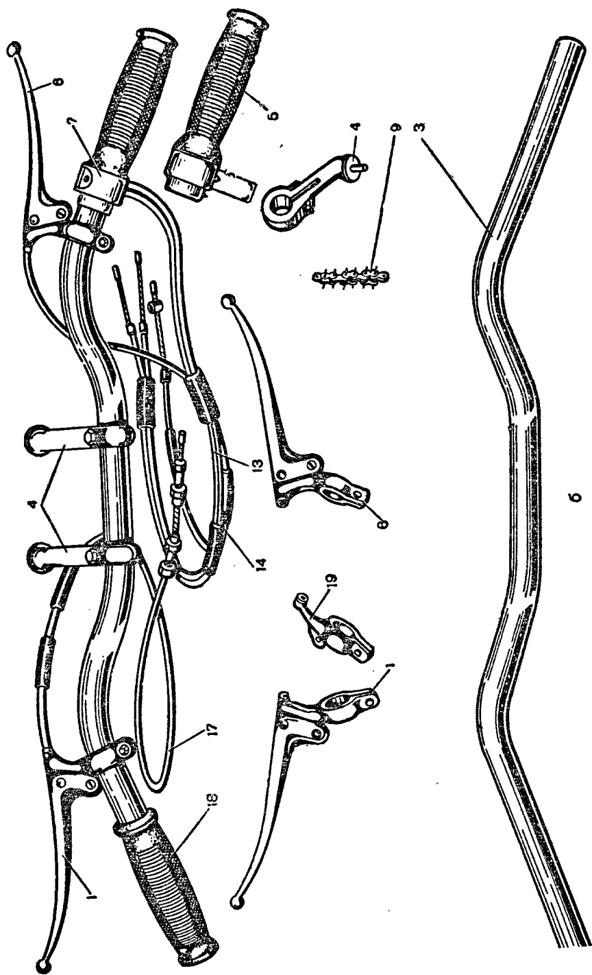
Рис. 9. Руль в сборе 2 — серий «Днепр»; 6 — серии «Урал»; 1 — рычаг сцепления; 2 — комбинированный переключатель; 3 — труба руля; 4 — кронштейн руля; 5 — ручка управления дросселями; 6 — рычаг ручного тормоза; 7 — корпус ручки; 8 — крышка корпуса; 9 — цепочка в сборе; 10 — ползун; 11 — регулировочный винт; 12 — пружина; 13 — трос дросселя; 14 — трос тормоза на переднее колесо; 15 — скоба троса; 16 — трос опережения зажигания; 17 — трос сцепления; 18 — рукоятка руля; 19 — основание рычага
