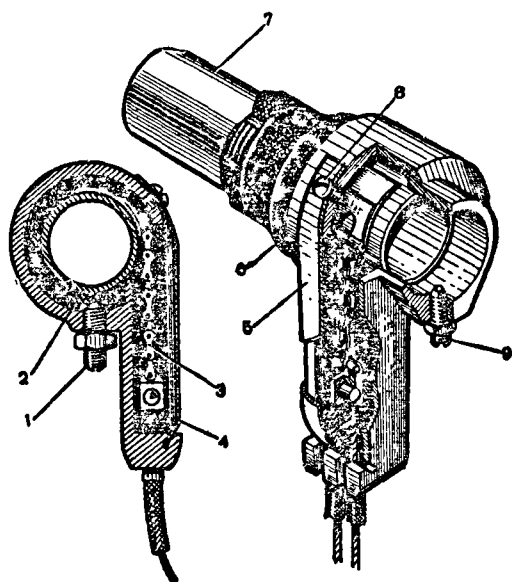
Рис. 10. Ручка управления дросселями катушечного типа:
