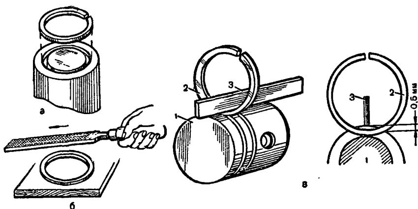
Рис. 14. Крепление поршневых колец при спиливании высоты их напильником: а — в пазу болванки; б — на доске укрепленного гвоздями; в — проверка поршневого кольца по глубине канавки в поршне; 1 — поршень; 2 — поршневое кольцо; 3 — линейка
