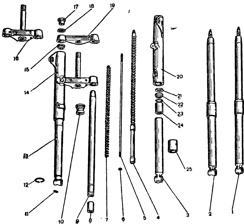
Рис. 61. Передняя вилка в разобранном виде:
