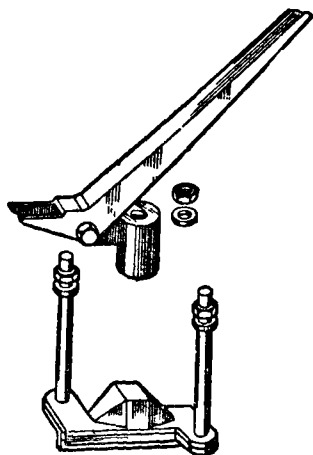
39. Приспособление для снятия пружин клапана
