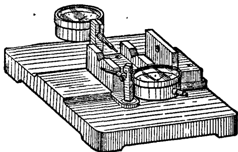
44. Приспособление для проверки бнения фаски головки клапана и стержня
