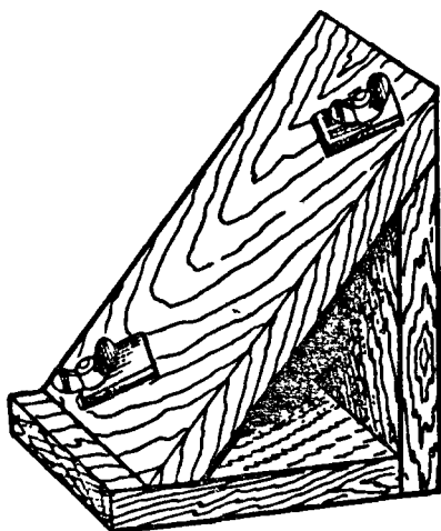
40. Приспособление для крепления головки цилиндра при обработке седел клапанов
