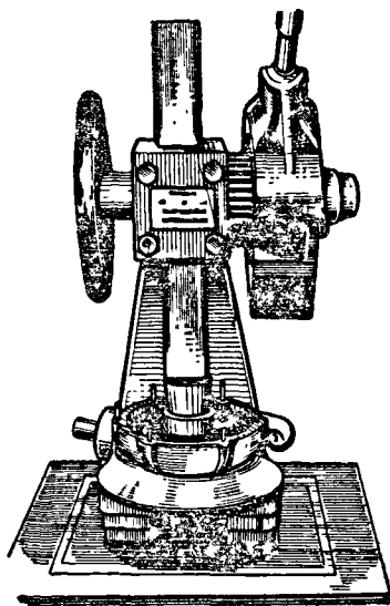
Р и с. 60. Запрессовка и выпрессовка деталей главной передачи
