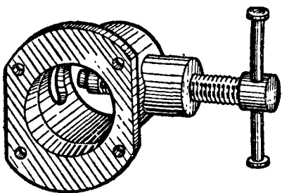
5. Приспособление для выпрессовки поршневого пальца
