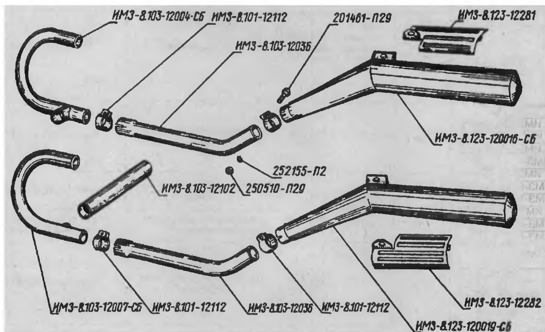
Выпускные трубы, глушители. Рис. 19-2
