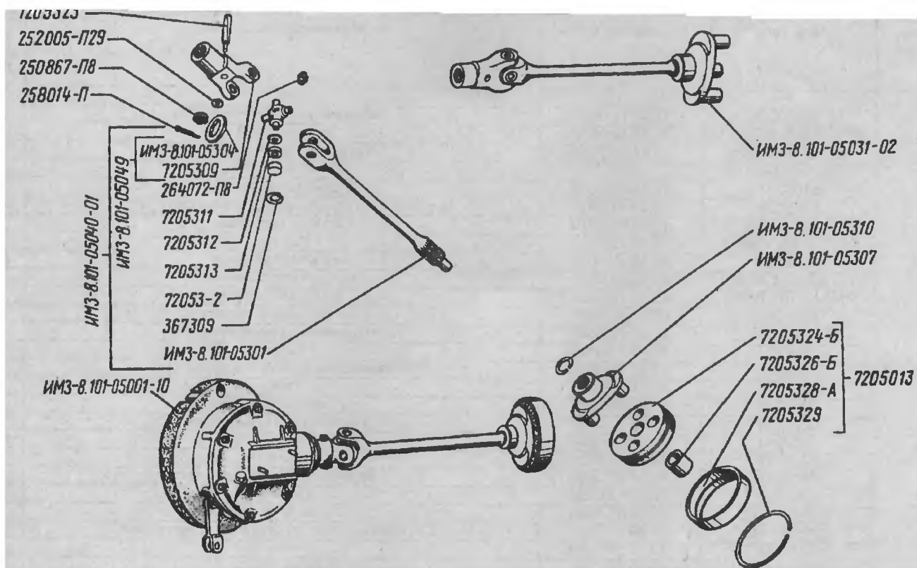
Главная передача, кардан. Рис. 16-1
