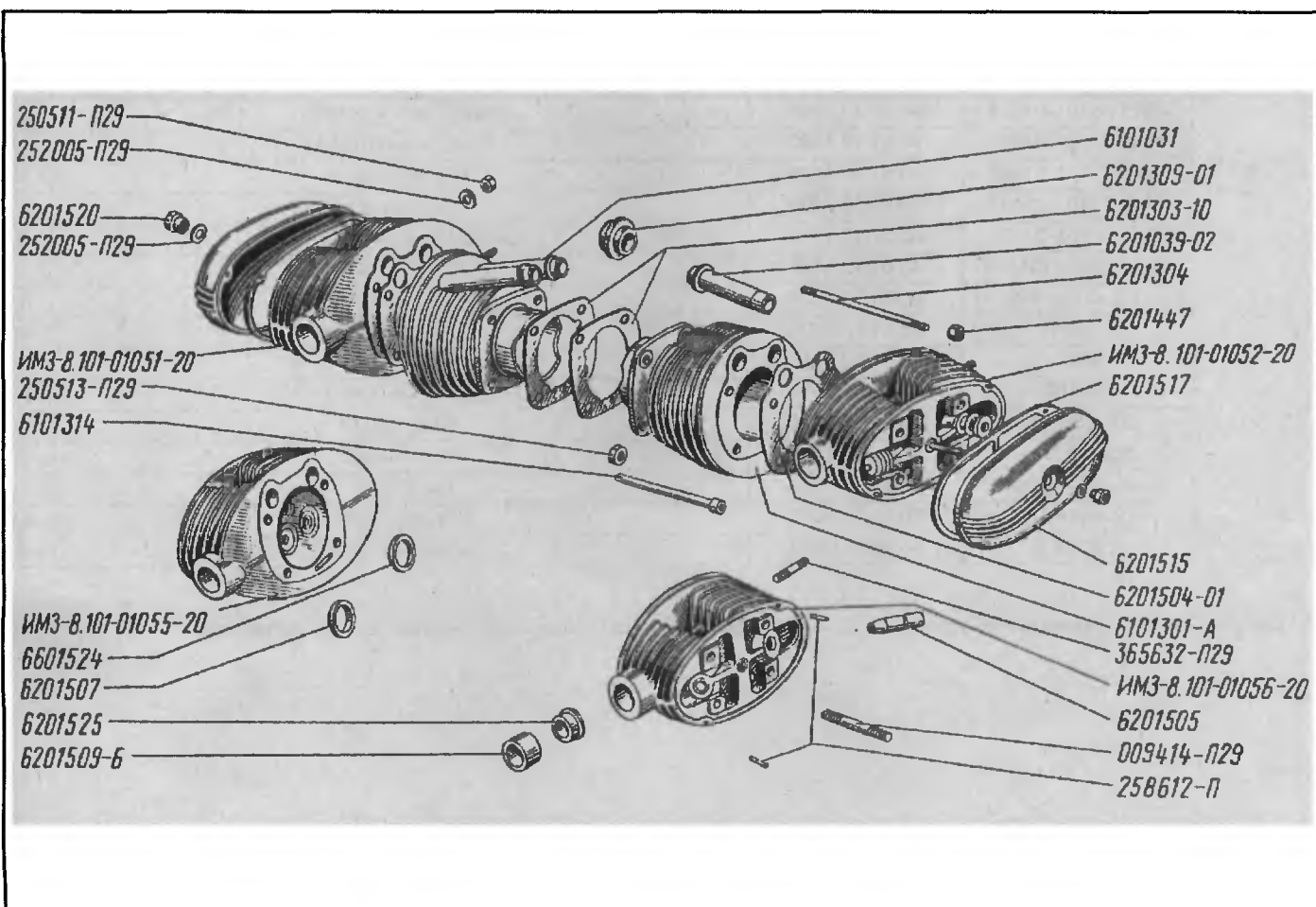
Цилиндры и головки цилиндров. Рис. 12
