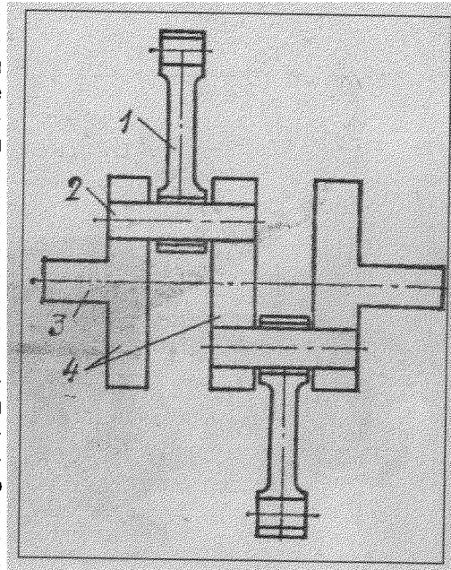
Рис. 5. Схема устройства кривошипно-шатунного механизма:
