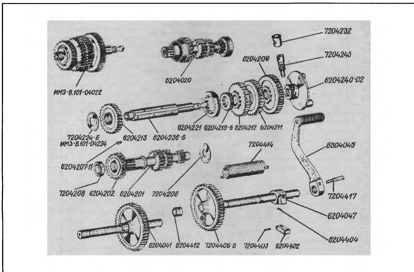
Валы и шестерни коробки передач. Рис. 6
