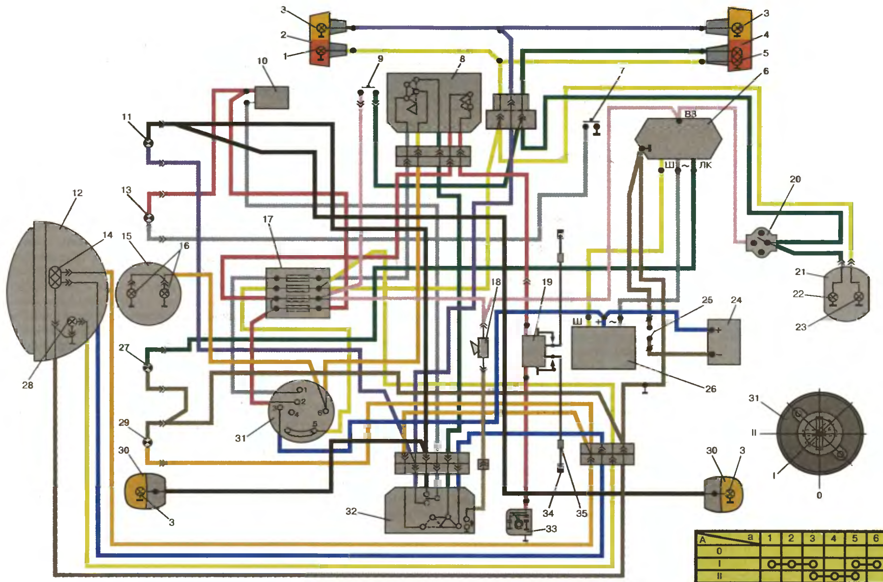
Схема электрооборудования мотоцикла ИМЗ-8.103-10:
