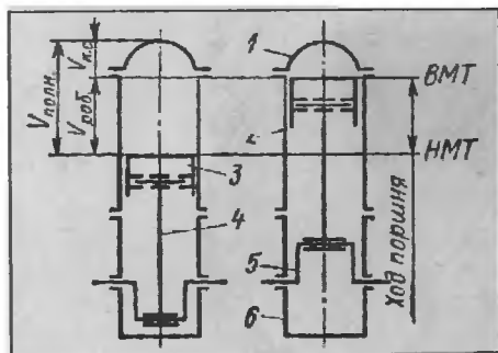
Рис. 1. Схема устройства четырехтактного двигателя:
