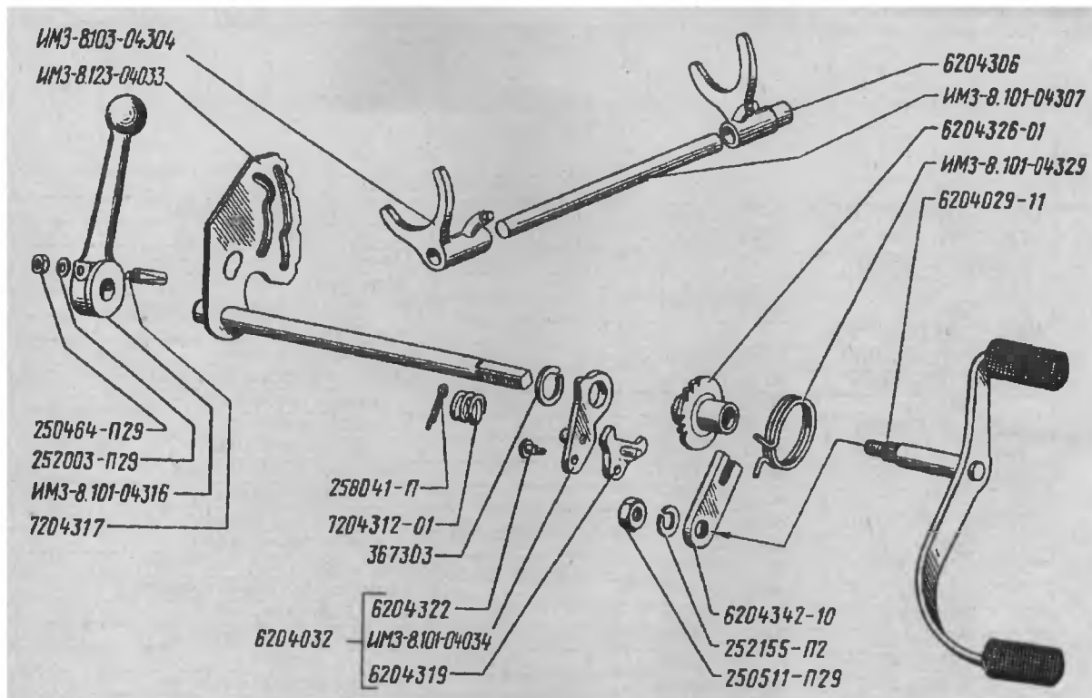
Механизм переключения передач. Рис. 15
