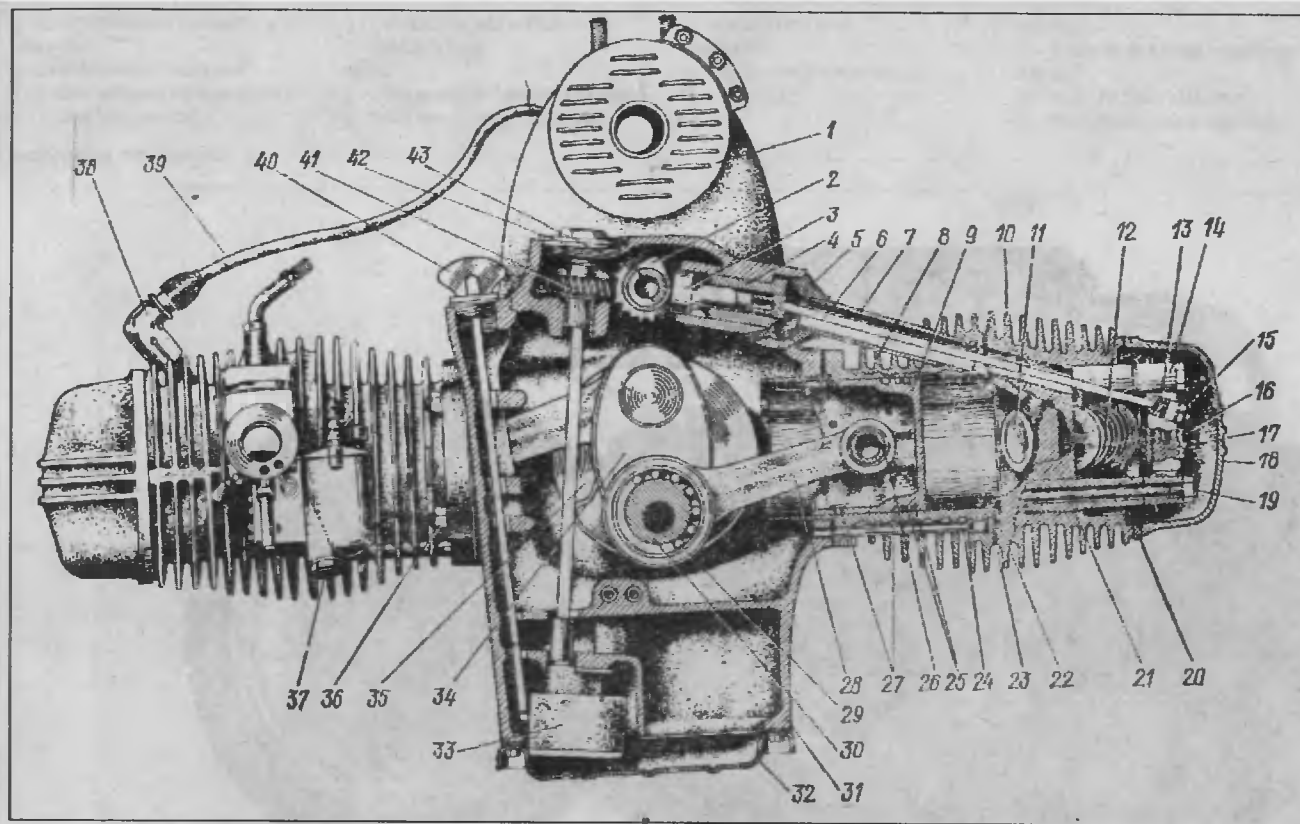
Рис. 3. Двигатель (поперечный разрез):
