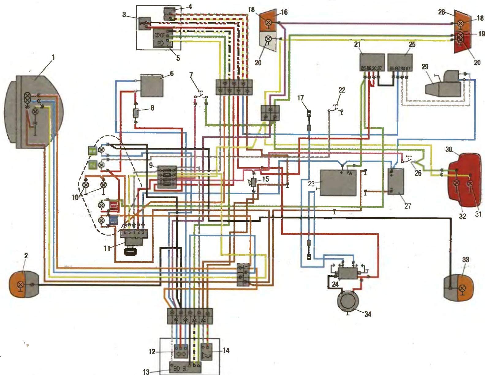
Схема электрооборудования мотоцикла ИМЗ-8.Т037 и его модификаций (включая мотоциклы с приводом на колесо коляски):
