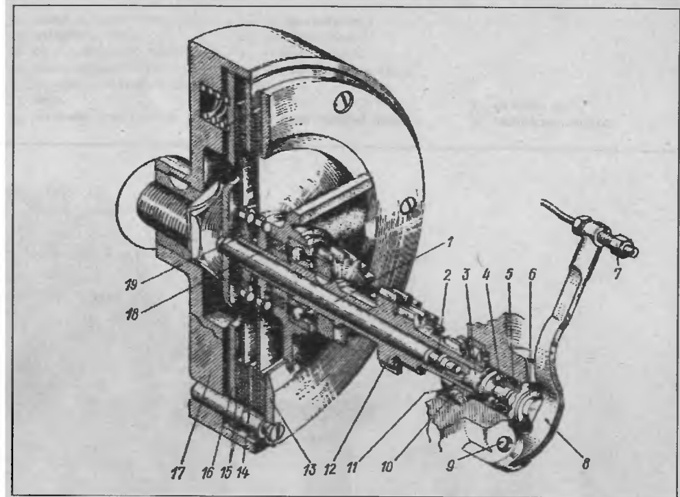
Рис. 8. Сцепление:
