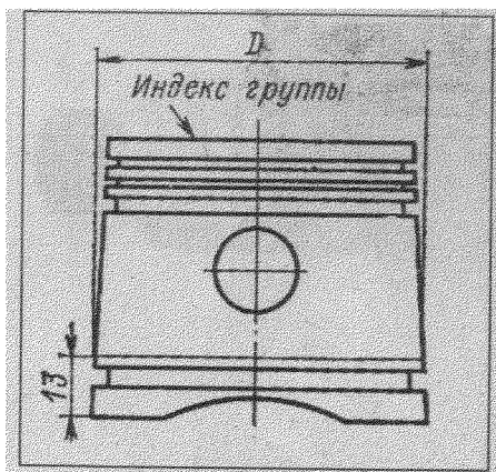
Рис. 4. Маркировка поршня
