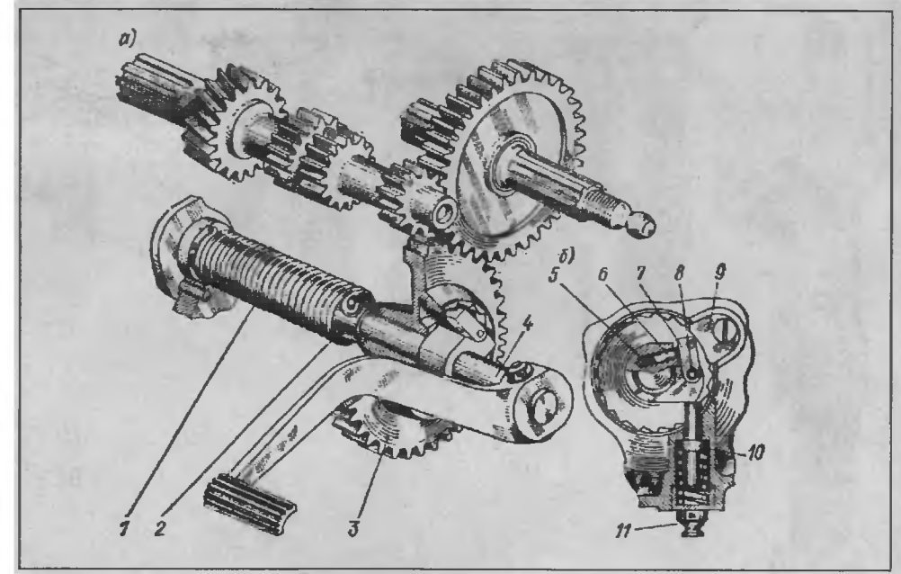
Рис.10. Пусковой механизм:
